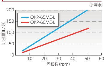
回転数-吐出量特性表
