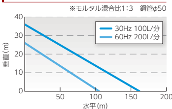
輸送距離(水平-垂直)特性表 OKP-65ME-L
