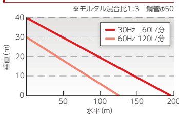
輸送距離(水平-垂直)特性表 OKP-60ME-L
