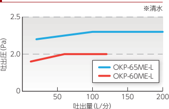
吐出量-吐出圧特性表
